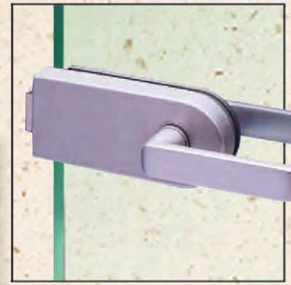
PL-DSR 2 9/16"H / 6 1/4" W
